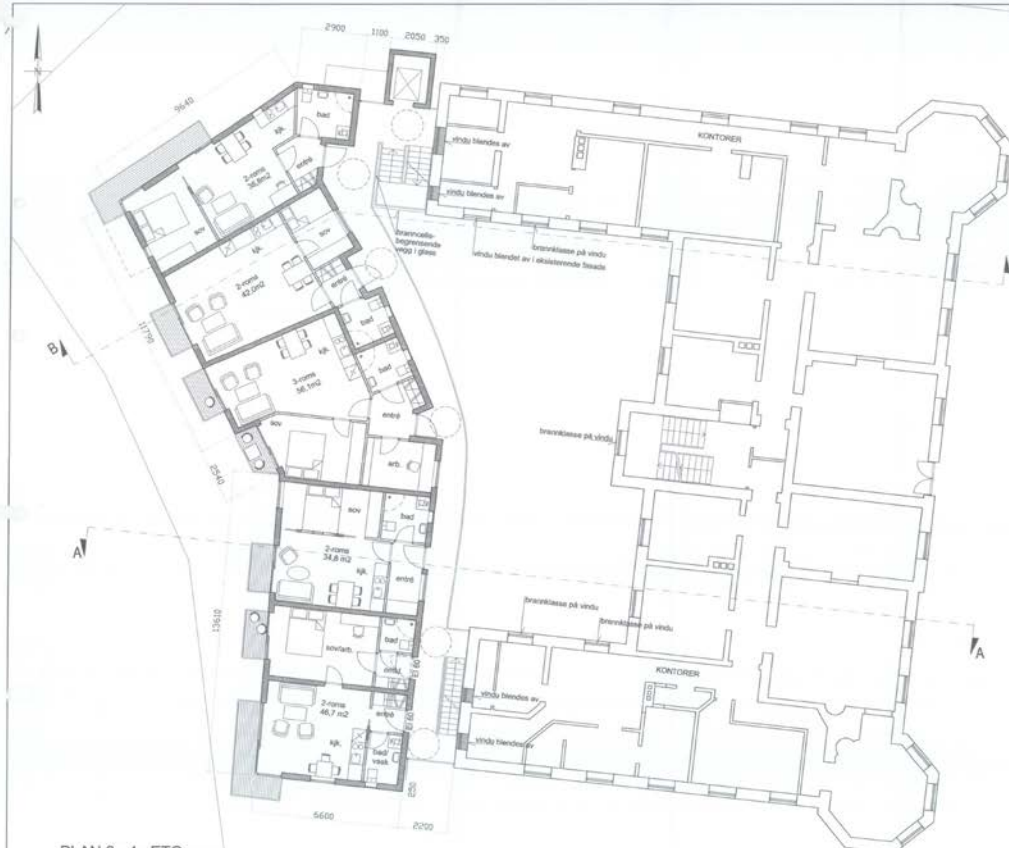
PLAN 2.- 4. ETG. BRA 260,0 m2
