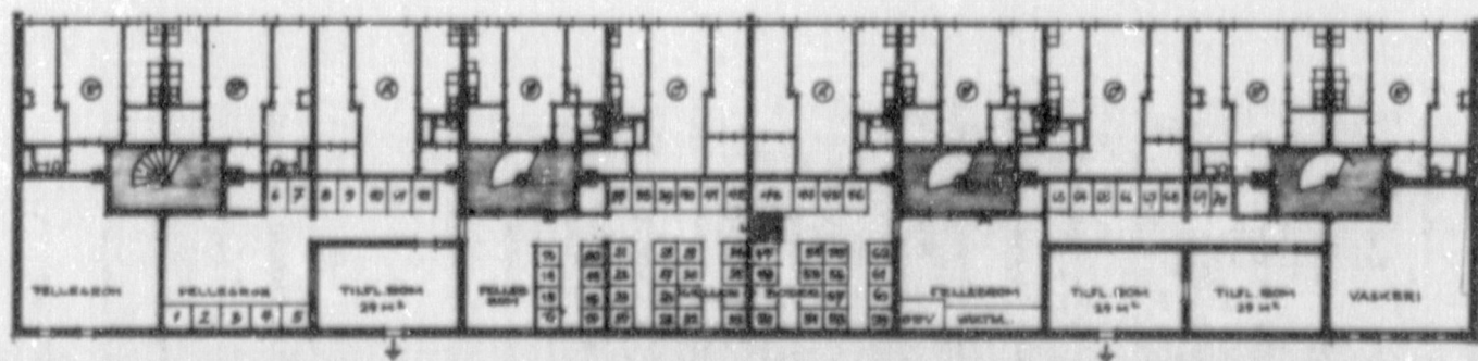
KJELLERPLAN
