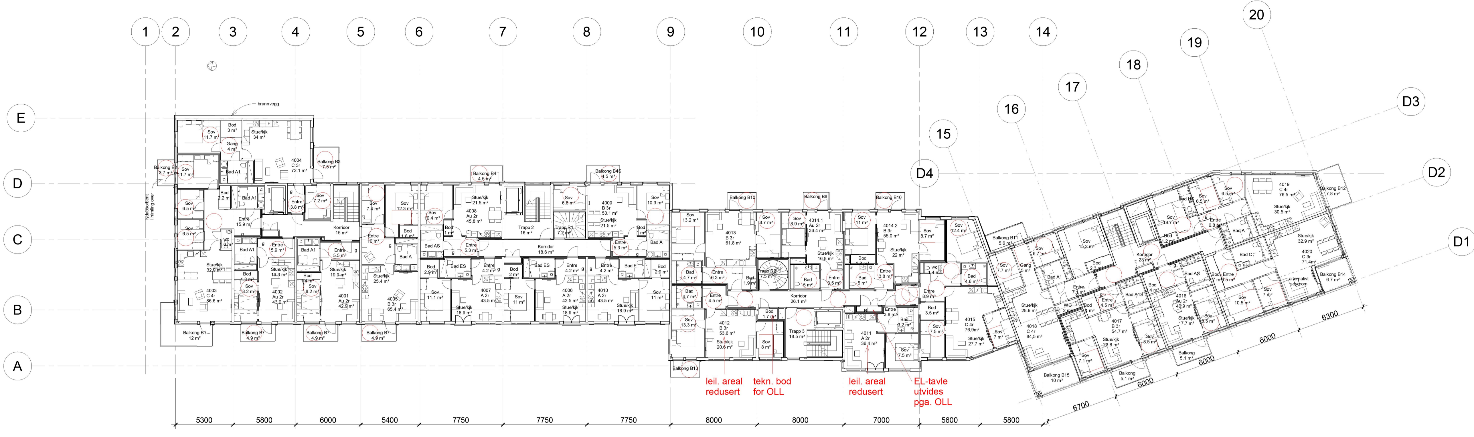
PLAN 4. ETASJE
