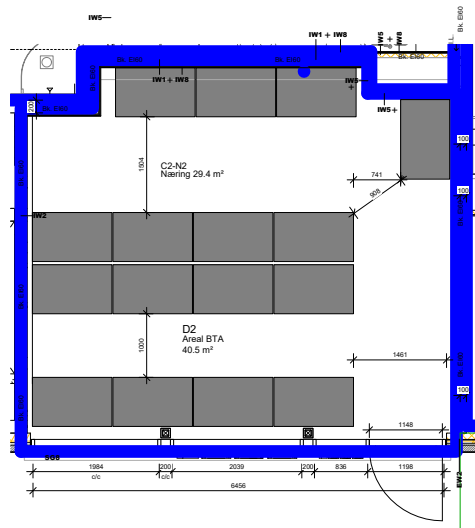
Næringslokale D2/N2 som avfallsrom - Alternativ 2 1 : 50
