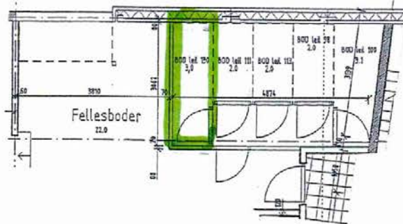
Plassering Byggetrinn 2 (1. etasje)
