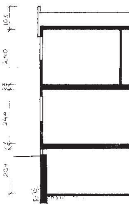
TVERR-SNITT
