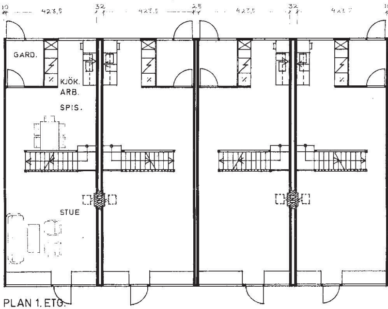
PLAN 1. ETG.
