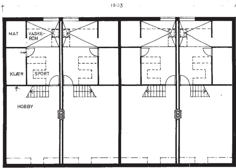
PLAN KJELLER
