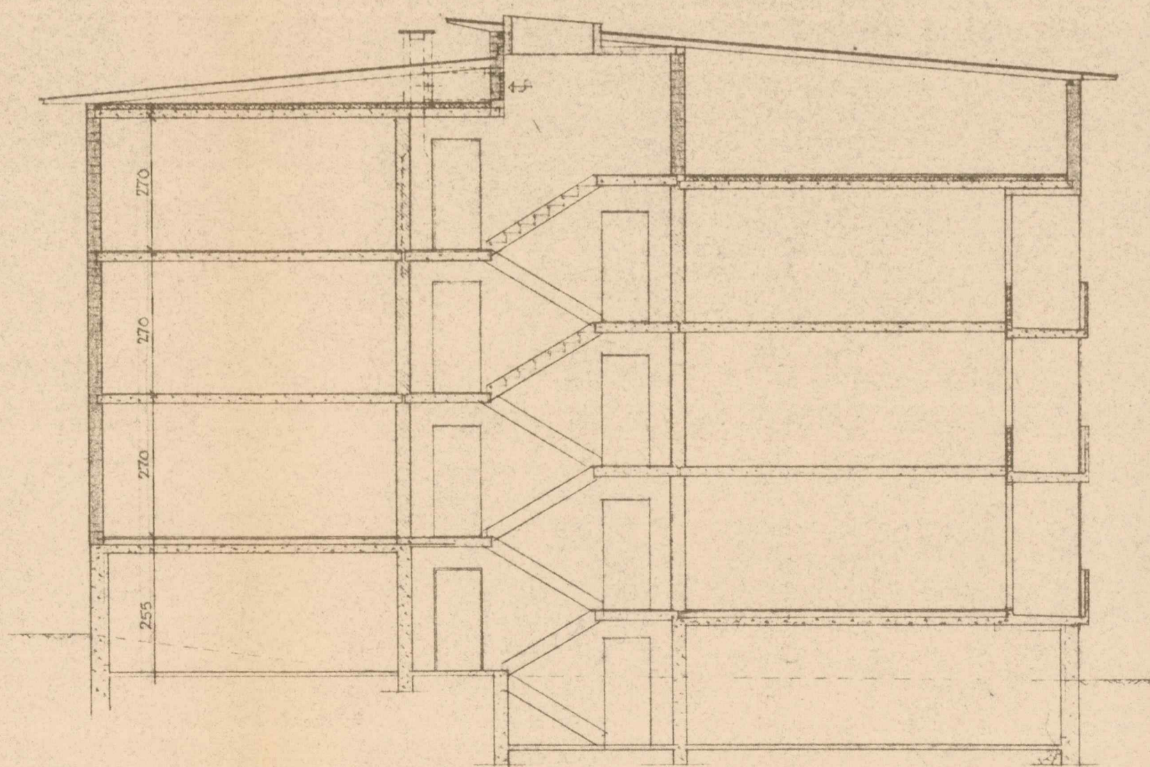
SNITT.
