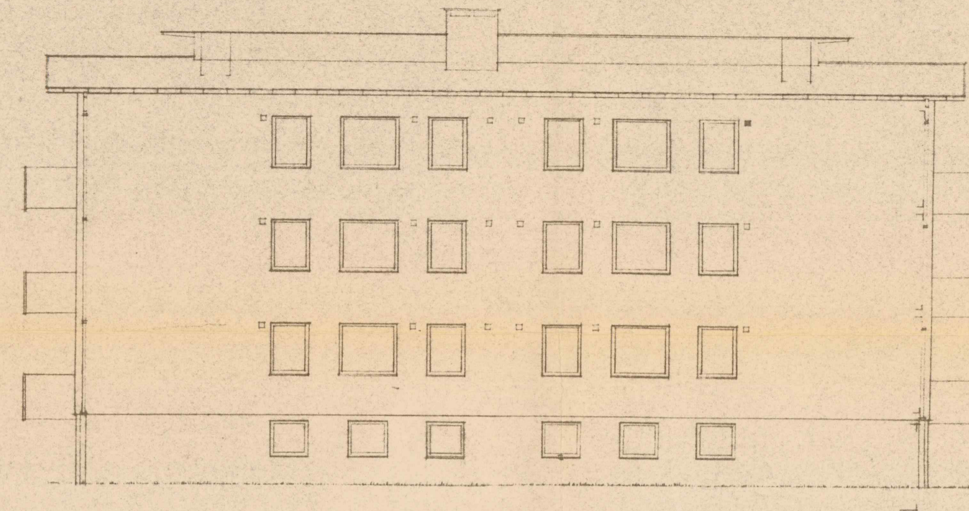
MOT NORD.
