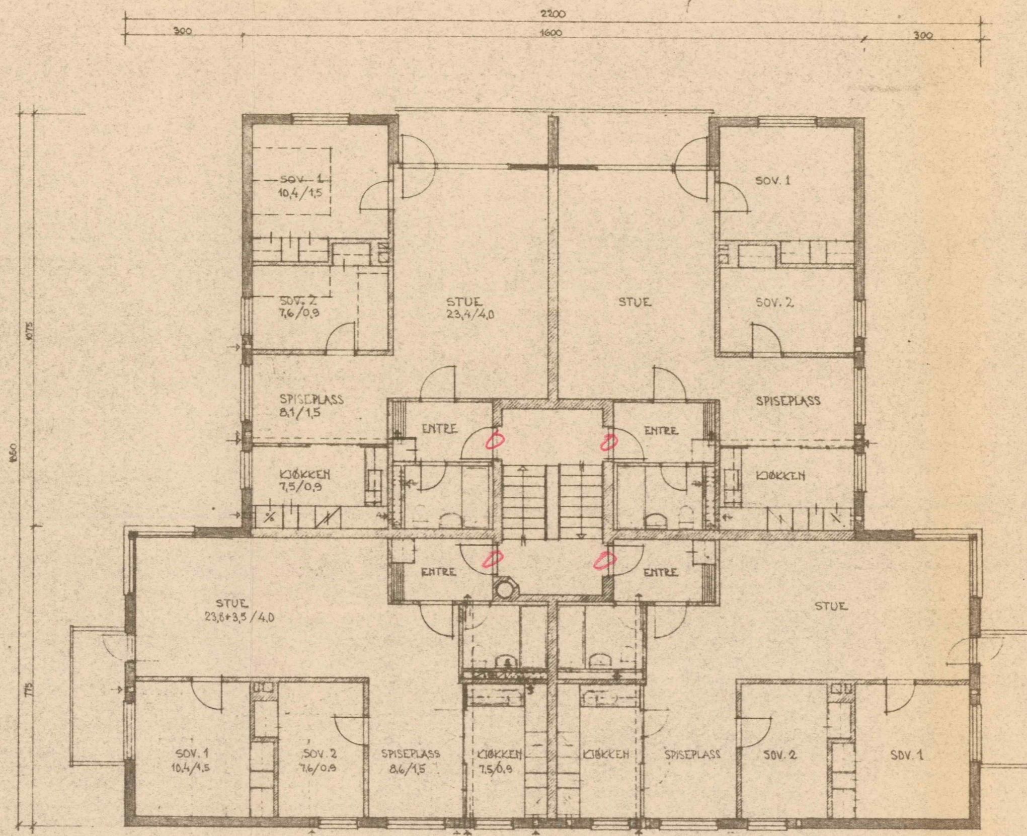
PLAN AV 1., 2. OG 3. ETASJE.
