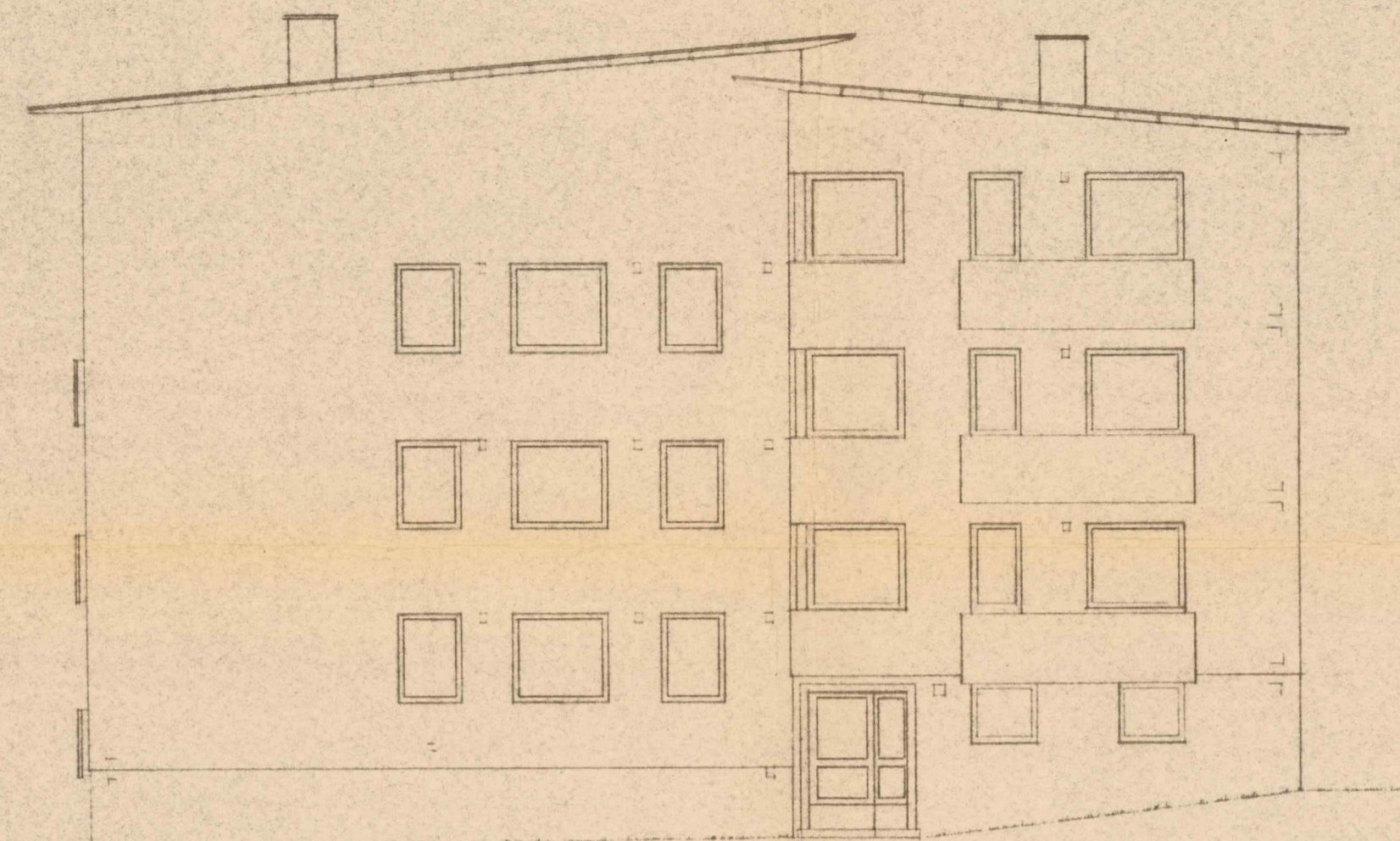
MOT ØST.
