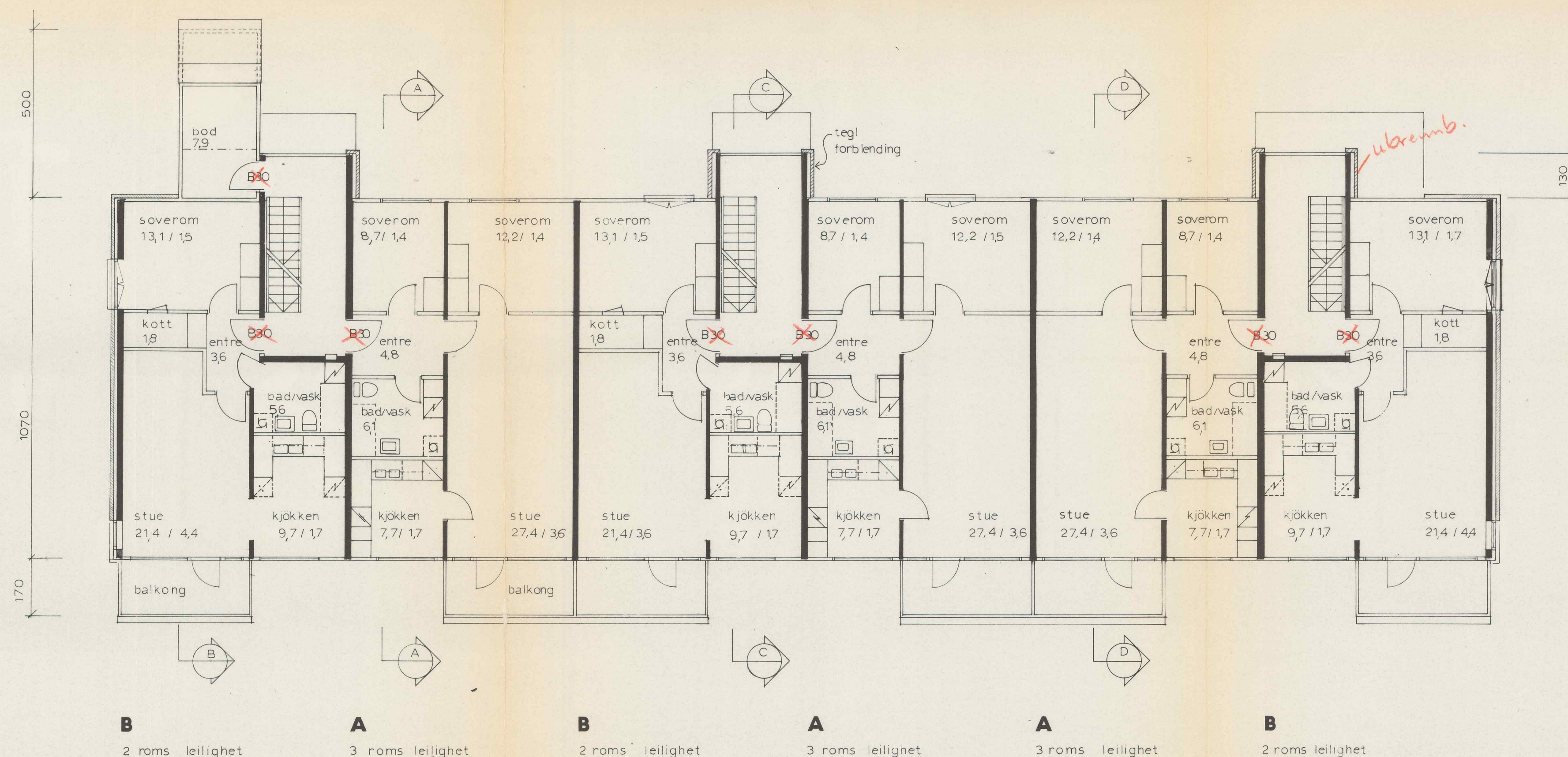
PLAN 2 ETASJE
