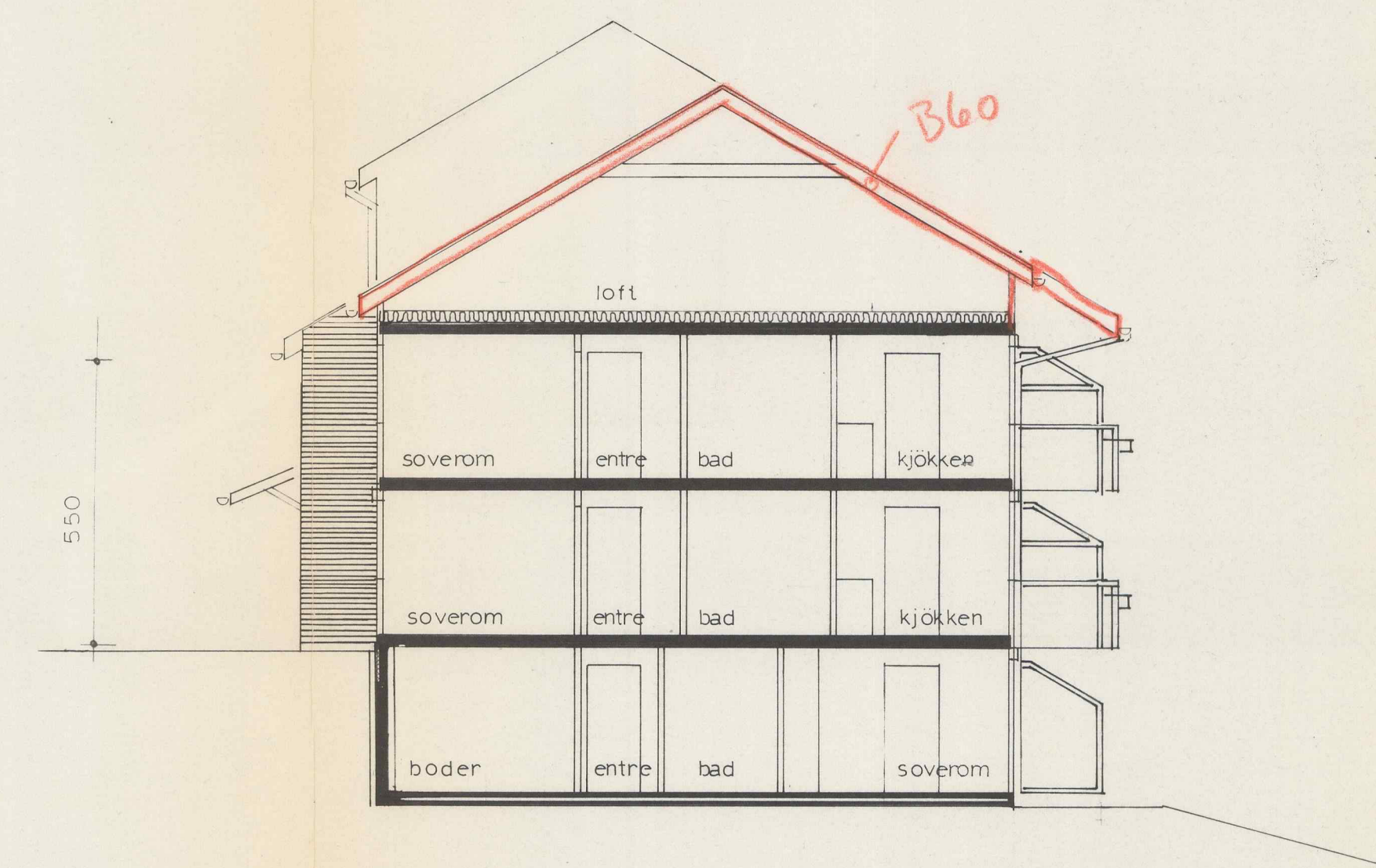
SNITT A-A
