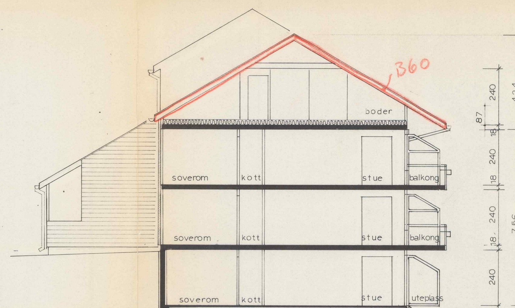
SNITT B-B
