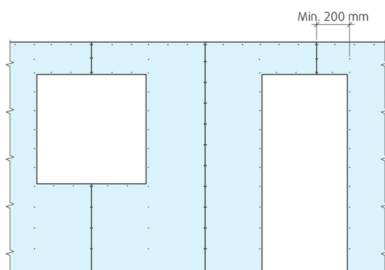
Fig. 46 Montering av plater ved dør- og vindusåpninger
