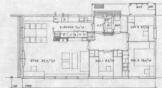
PLAN AV 1. ETASJE
