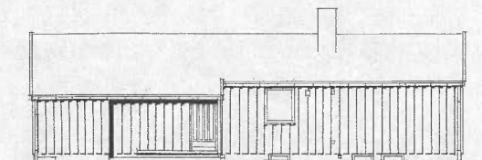
FASADE MOT NORD
