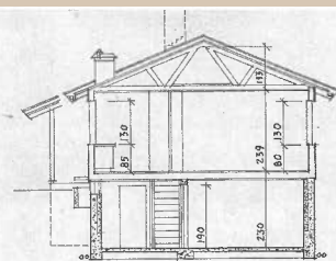
SNITT
