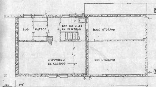
PLAN AV KJELLER
