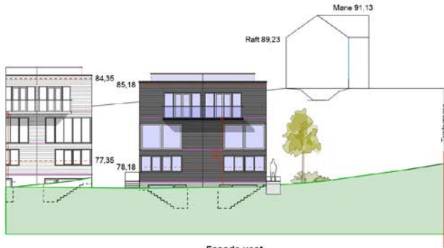
Fasade vest
