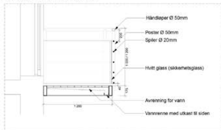
DETALJSNITT 1:20
