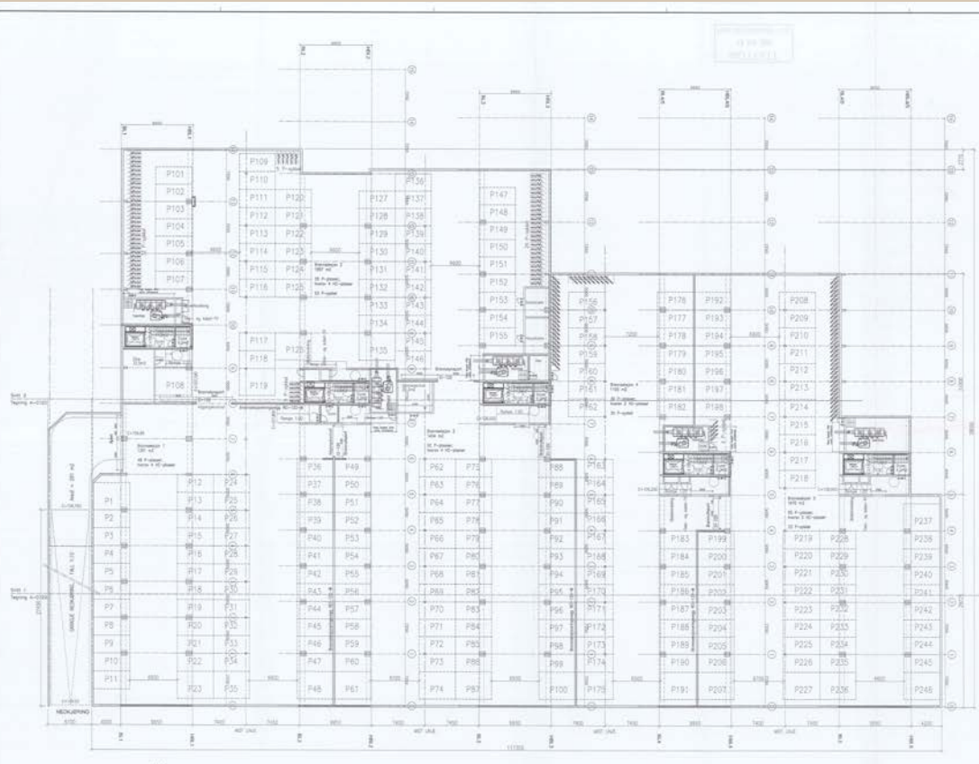
Plan garasje
