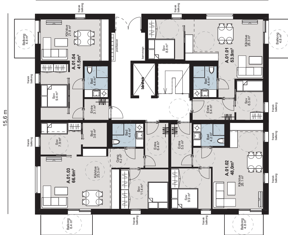
Bygg A - Plan 01 1:100
