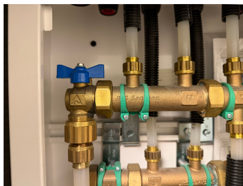
Stoppekrane i rør i rør skap.
