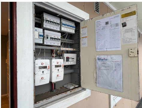
Sikringsskap i yttervegg. Utvendig adkomst.
