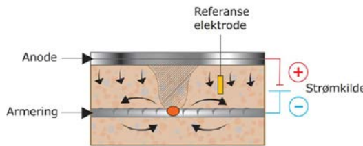
Illustrasjon katodisk beskyttelse
