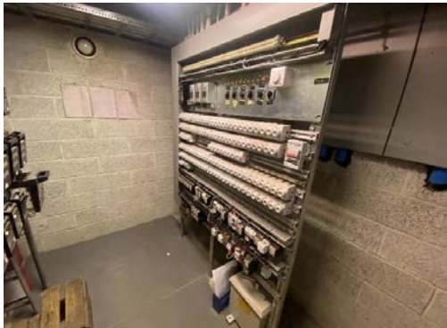
Hovedtavle med skrusikringer og berøringsfare
