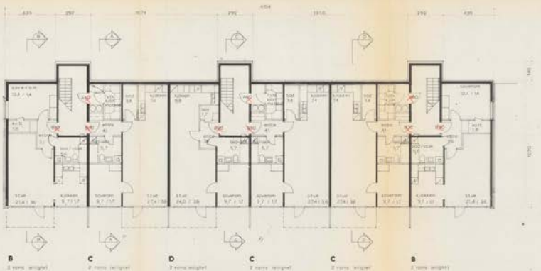
PLAN UNDERETASJE
