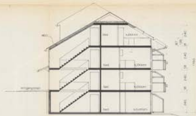
SNITT C-C
