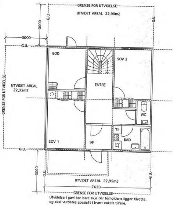
PLAN 1. ETASJE
