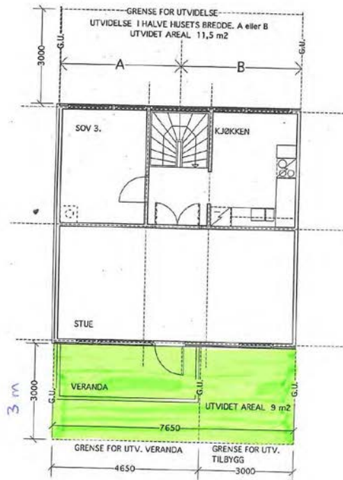
PLAN 2. ETASJE
