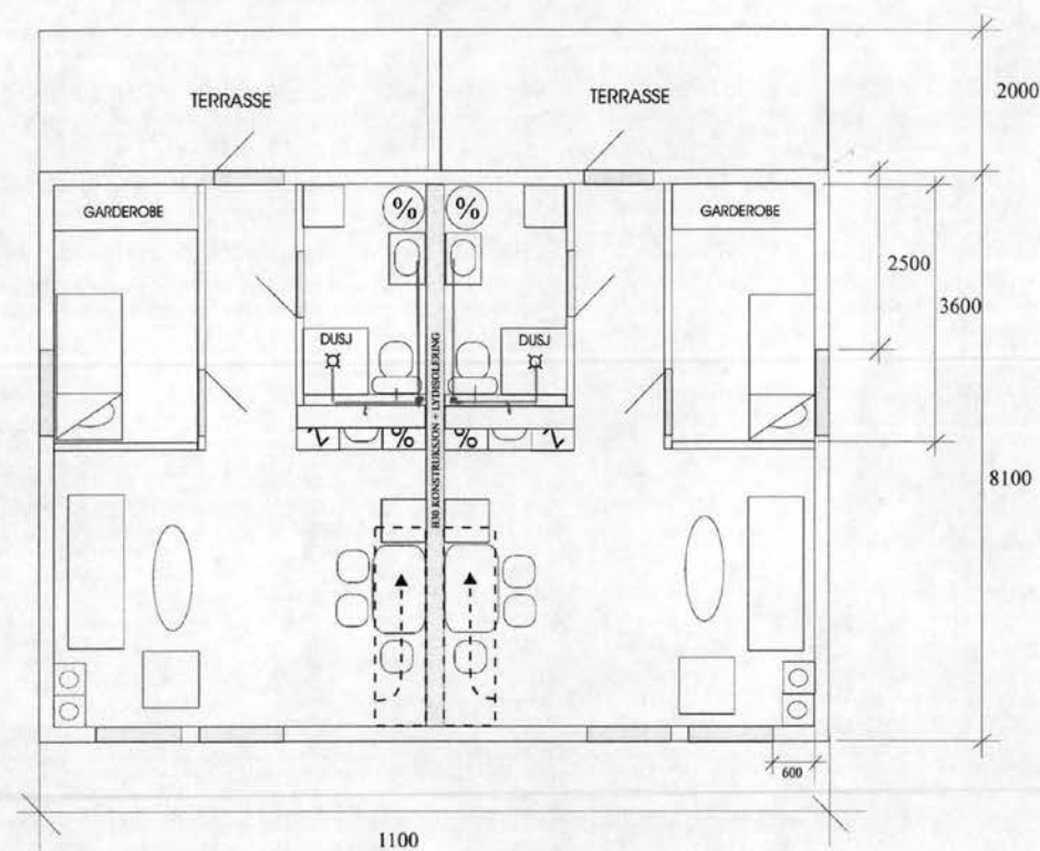
PLAN 1-ETG 201\684
