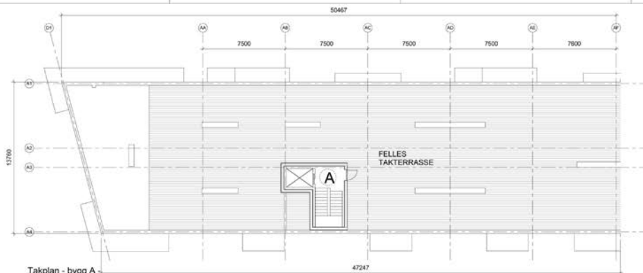
2 Takplan - bygg A - rammesøk 1:150
