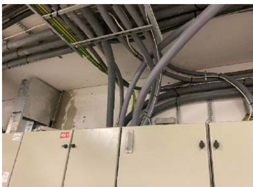
Inntakskabler, stigeledninger og hovedtavle
