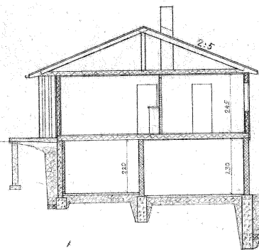
Snitt
