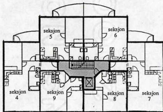
Rathkesgate 3, Plan 2.etg., Seksjon 4-9
