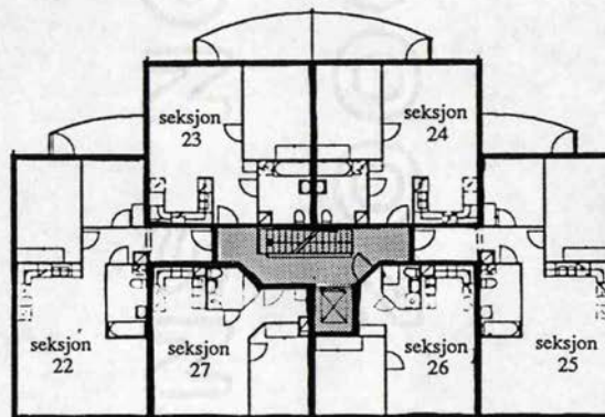
Rathkesgate 3, Plan 5.etg., Seksjon 22-27
