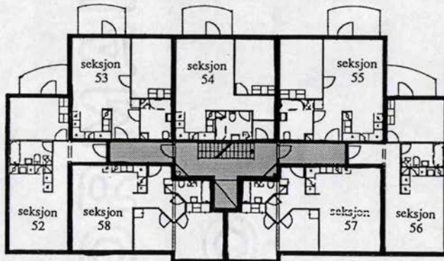
Rathkesgate 6, Plan 5.etg., Seksjon 52-58
