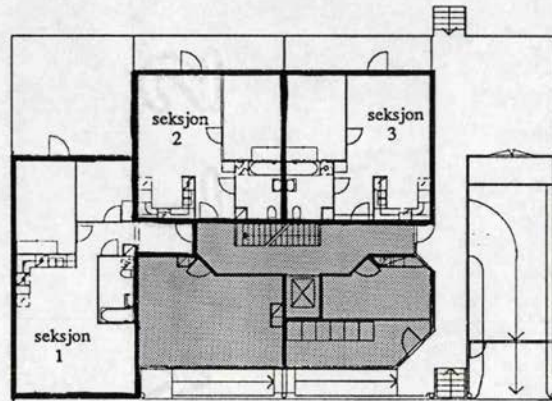
Rathkesgate 3, Plan 1.etg., Seksjon 1-3
