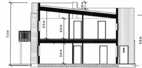
Snitt A-A
