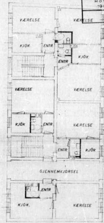
1. etasje etter forandring
