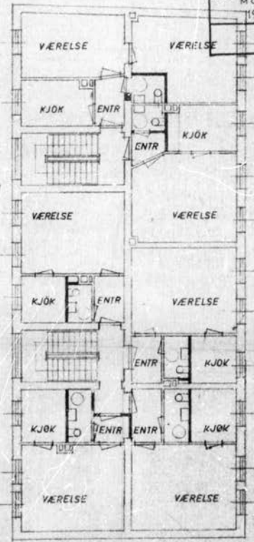
2, 3 og 4 etasje etter forandring DUNS gt. 4, bakbygningen, innredning og vannklosetter M: 1:100 OSLO 17/10 -72
