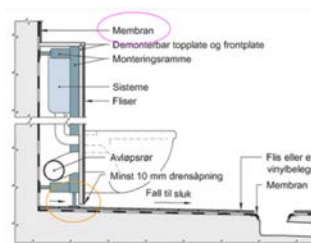
Fig. 63 Eksempel på løsning med installasjonvegg inne i vådrommet
